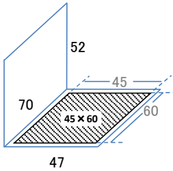
0.4m 3 ガス窯A
