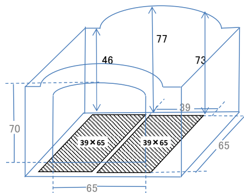
イッテコイ窯
