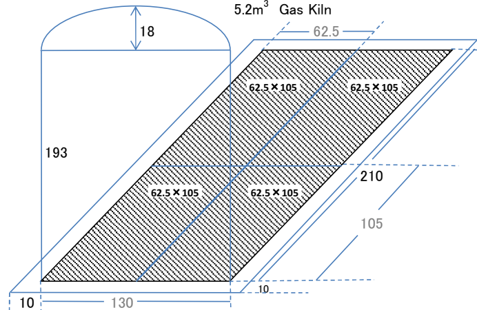
5.2m 3 ガス窯
